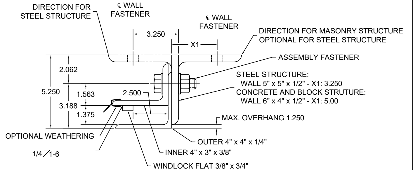
GUIDE ASSEMBLY TYPE DC 6 SCALE: 3" = 1'-0"
