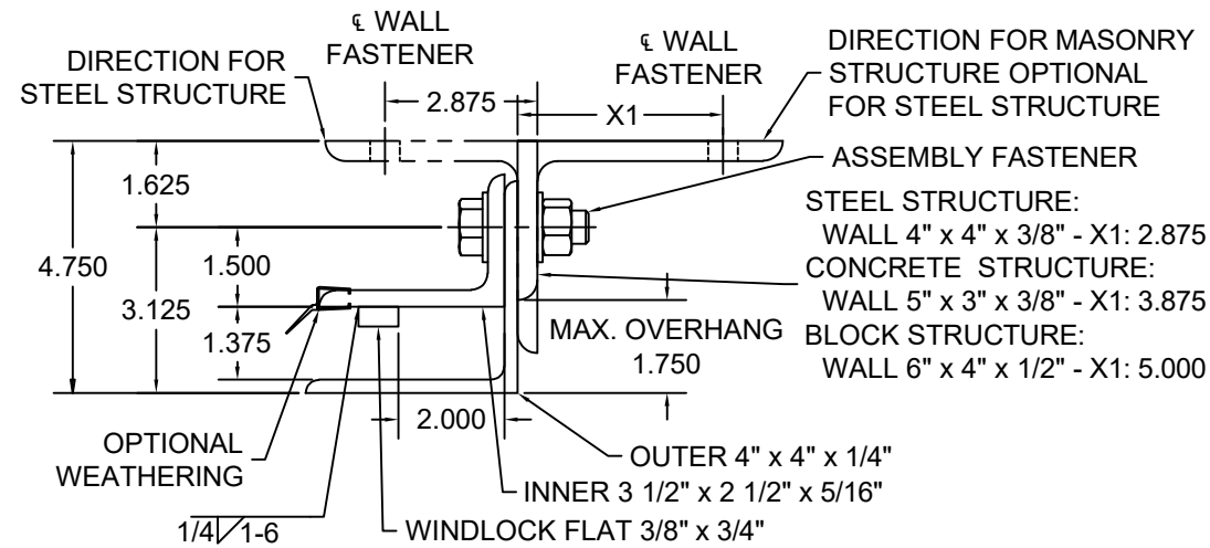
GUIDE ASSEMBLY TYPE DC 5 SCALE: 3" = 1'-0"
